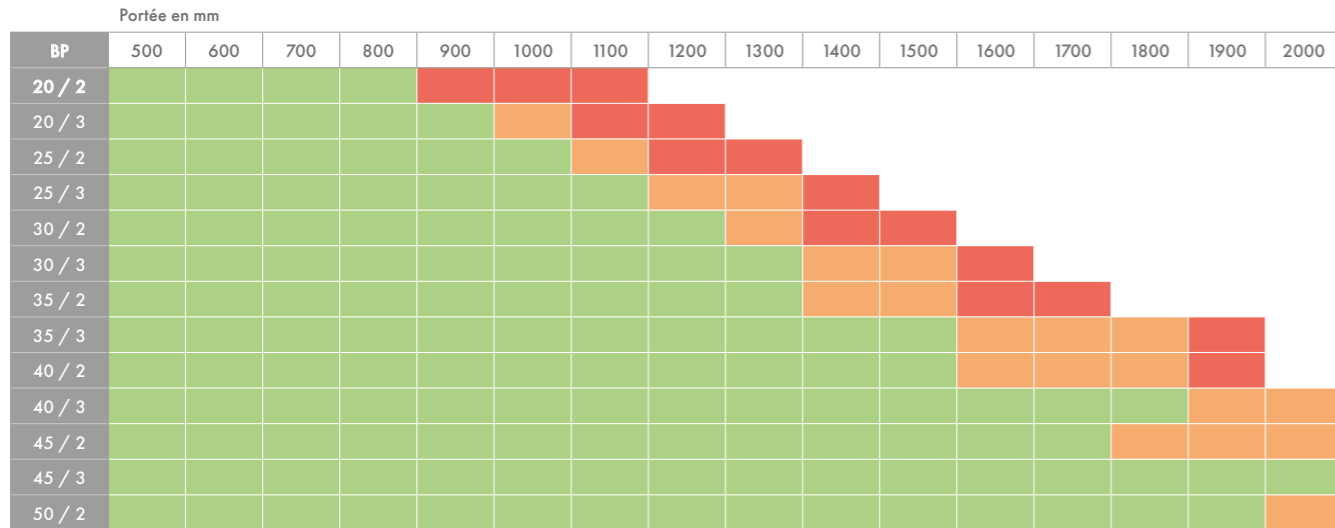
MAILLE DE 30 x ...
