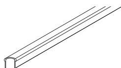
MAIN COURANTE Dimensions (l x h) : 69 x 62 mm. Longueur : 6000 mm.
