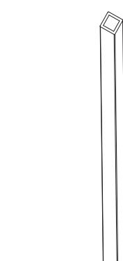
POTEAU Dimensions (l x h) : 50 x 50 x 7,5 mm. Longueur : 6000 mm.
